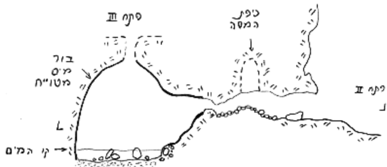
חתך אורך e-e'
