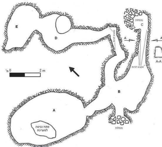
איור 3: תכנית וחתך מערכת המסתור בחורבת זבדה (שרטוט: ד' רביב וא' טבגר)
