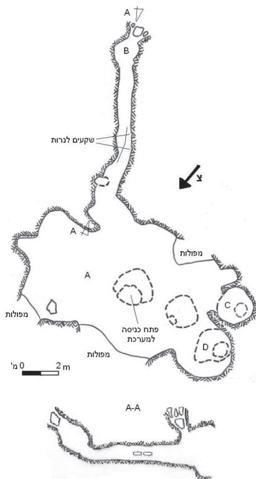
איור 12: תכנית וחתך מערכת המסתור בחורבת עררה (שרטוט: ד' רביב וע' עבאדי)
