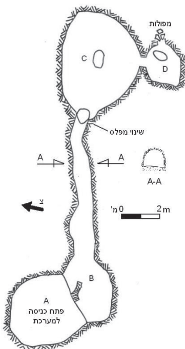
איור 7: תכנית וחתך מערכת המסתור בחורבת חנונה (שרטוט: ד' רביב וא' טבגר)
