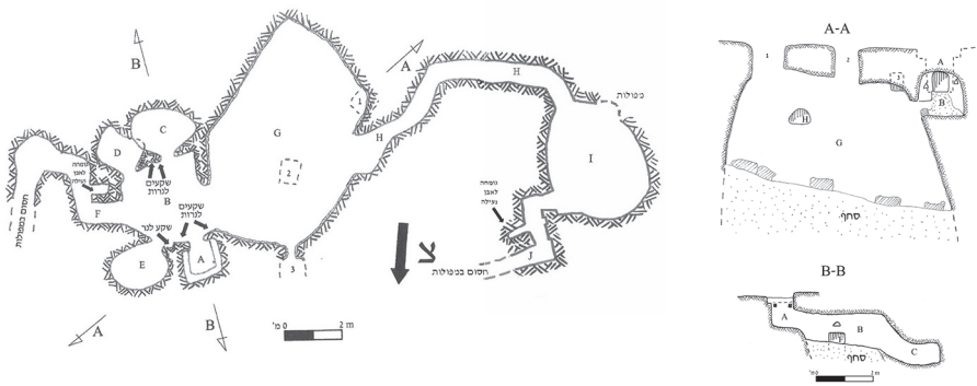
איור 5: תכנית וחתך של מערכת המסתור בחורבת א־דככין, כוללת האגף "החדש" (שרטוט: א' קליין וד' רביב)
